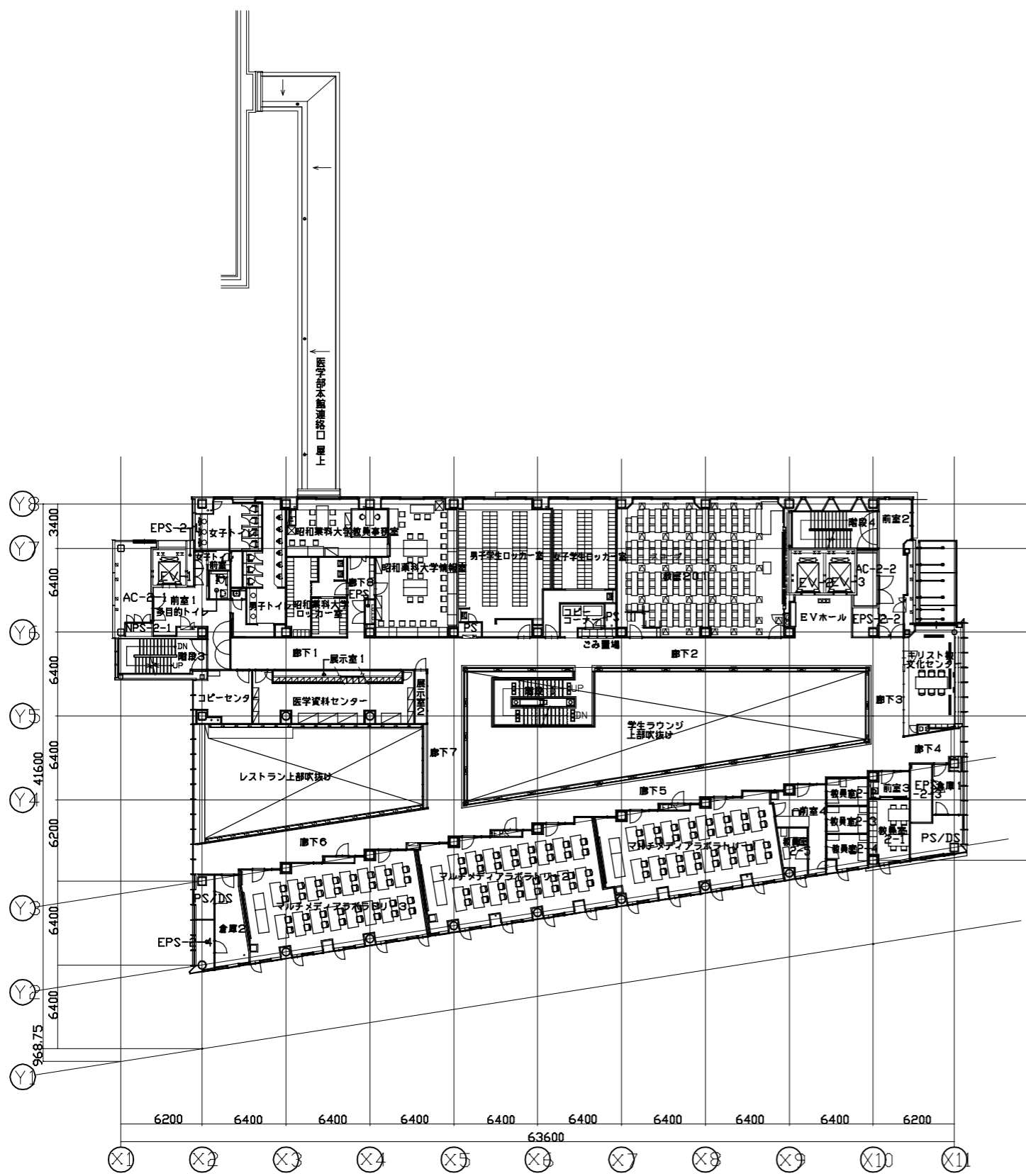
2階平面図
