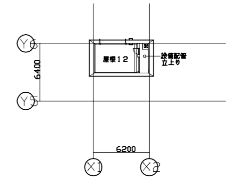
RF階平面図
