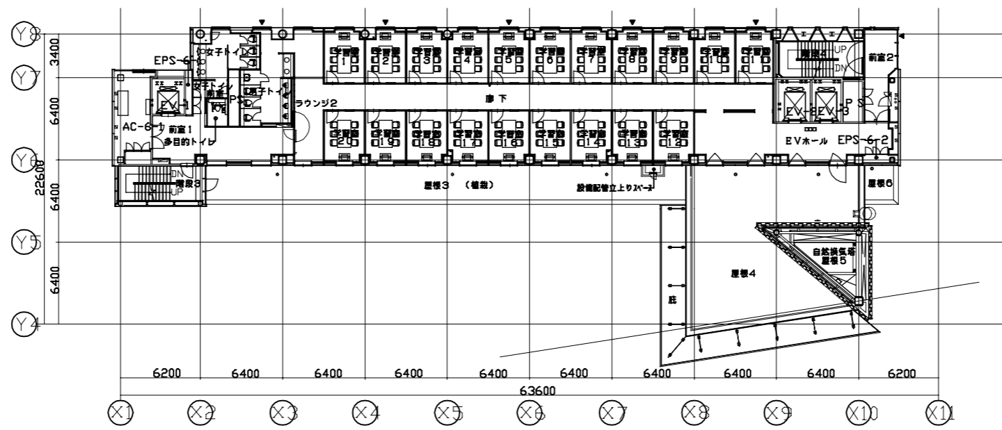
6階平面図
