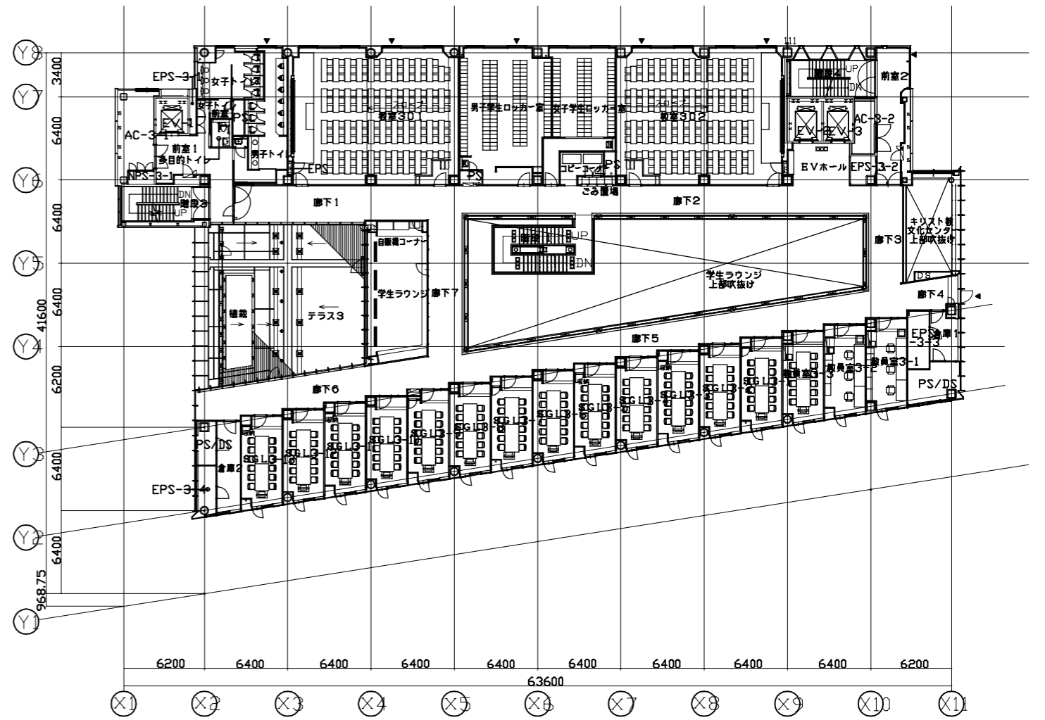
3階平面図
