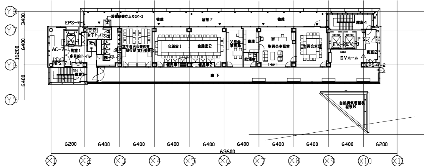
7階平面図
