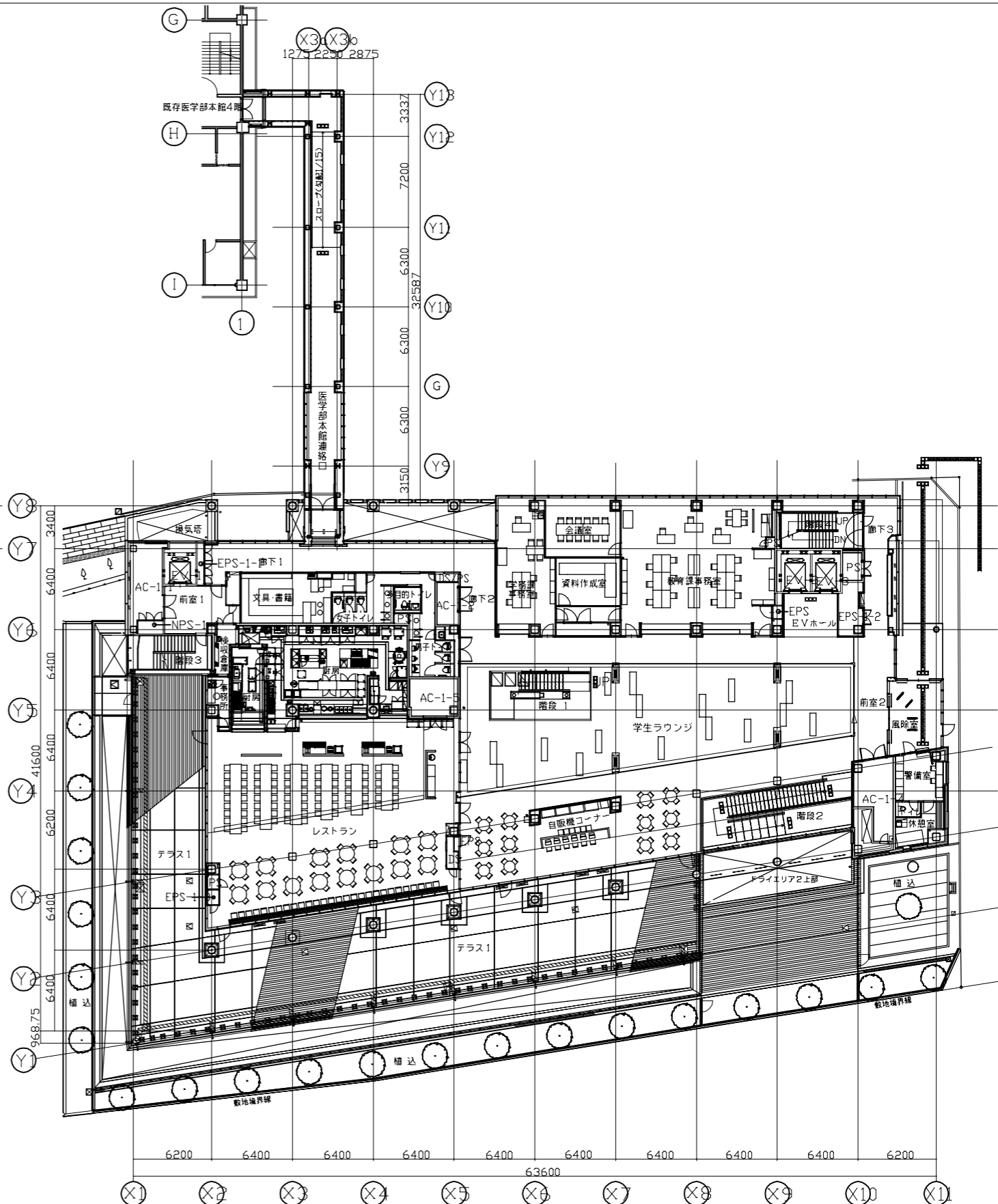
1階平面図
