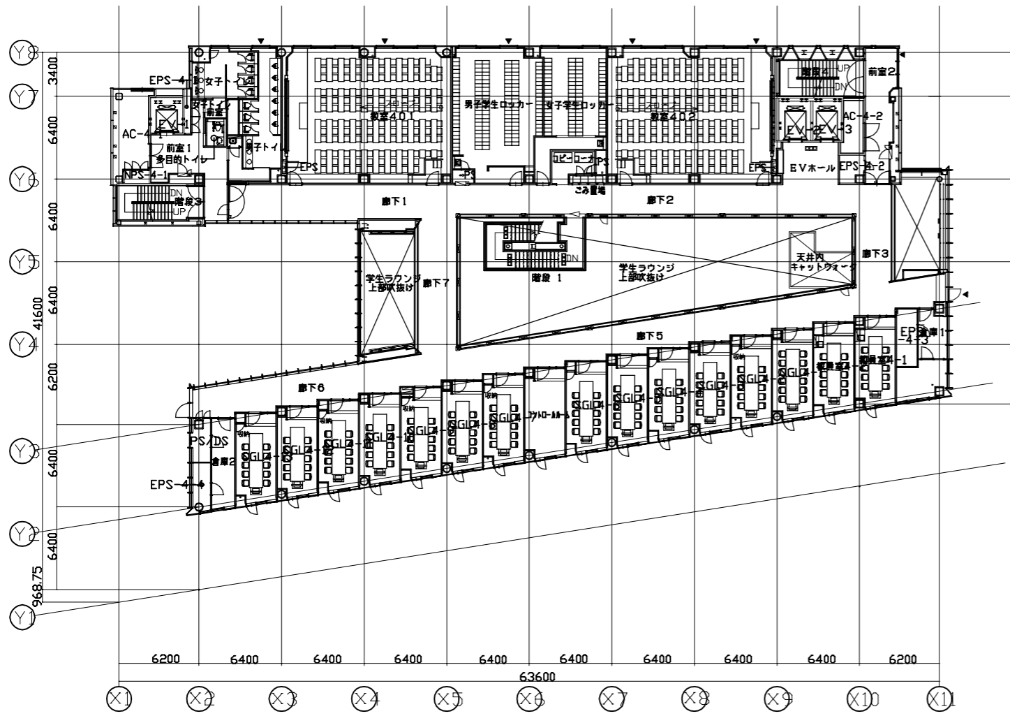
4階平面図
