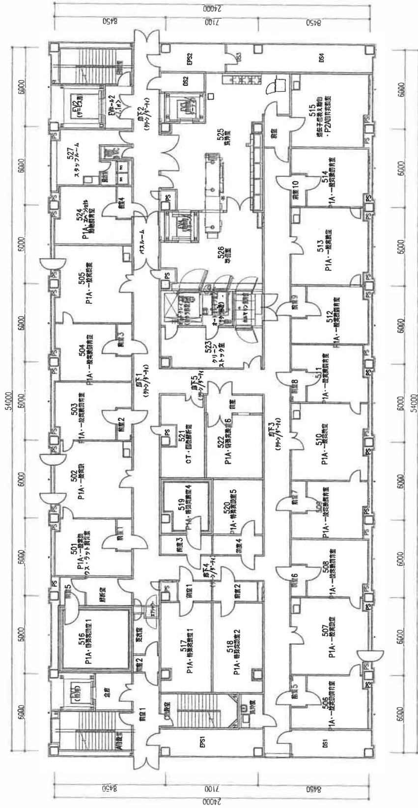
校地校舎等の図面-31
