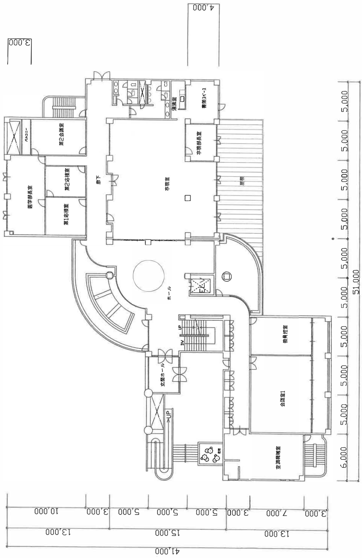
校地校舎等の図面-8
