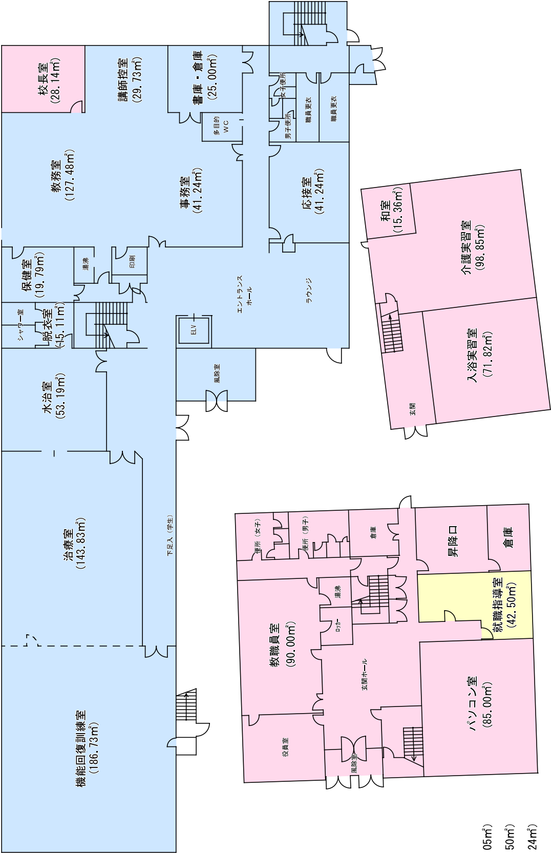
本部棟・既存棟（1）・既存棟（2） 1階平面図
