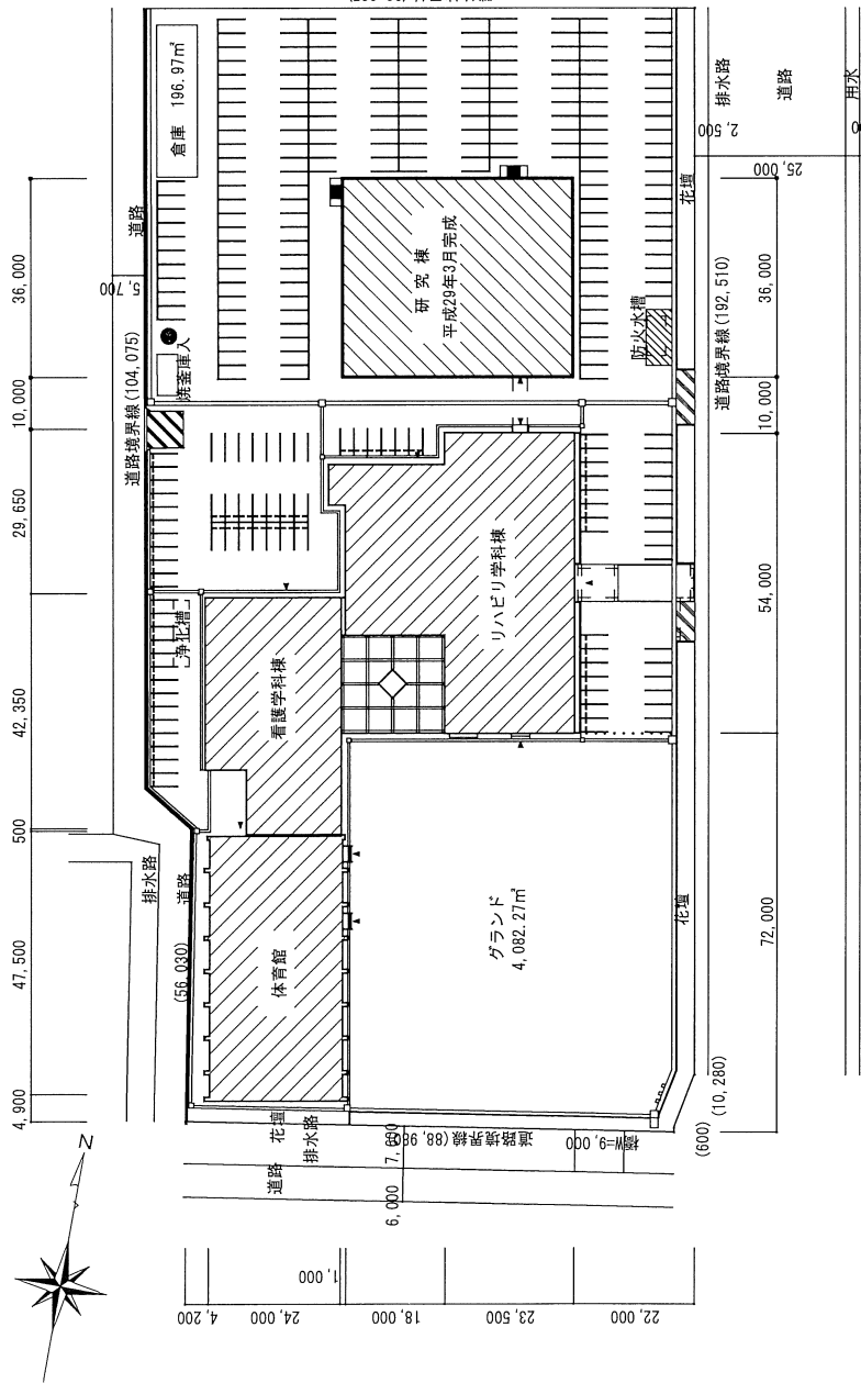
敷地面積 19,644.44㎡ 地名地番: 福井市江上町55字鳥町13番1 配置図 1/1500
